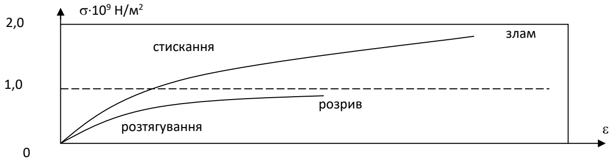
Рис. 2. Діаграма деформації для кістки
