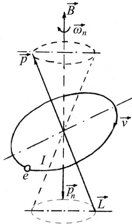
Рис. 2.2. Прецесія електрону
