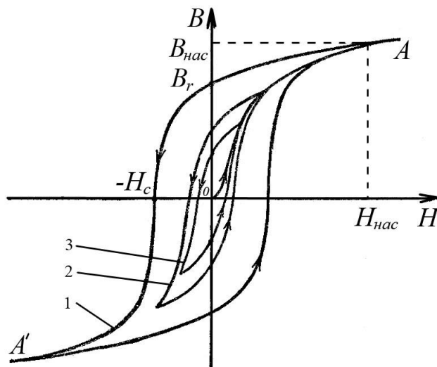
Рис.2.5. Петля гістерезису
